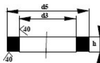
Kötőgyűrű „B”
